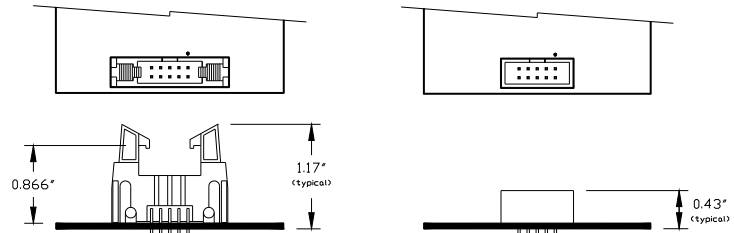
Long Ejectors
